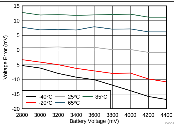
Figure 18. V_{\text{Err}} Across VIN (0 mA)
